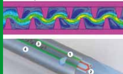
Tropfer-Labyrinth mit turbulentem, selbstreinigendem Fluss
